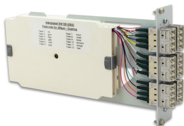
FO Splice Module Twin 7DU
