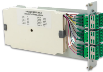
FO Splice Module Twin 7DU
